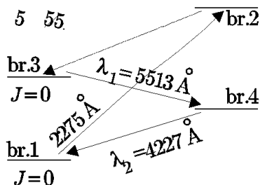
Slika 4.1: Kaskadna emisija atoma Ca .
