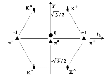
Slika 8.8: Hadronski K -supermultiplet.
