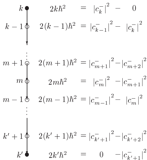
Slika A.3: Standardni bazis \mathcal{V}^{(k)} .
