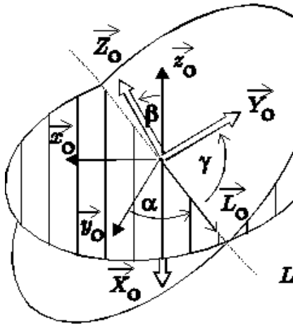
Slika 6.1: Euler-ovi uglovi: \alpha, \beta, \gamma . \{\mathbf{x}_0, \mathbf{y}_0, \mathbf{z}_0\} su ortovi prvog koordinatnog sistema, \{\mathbf{X}_0, \mathbf{Y}_0, \mathbf{Z}_0\} drugog; \mathbf{L}_0 je ort linije čvorova.
