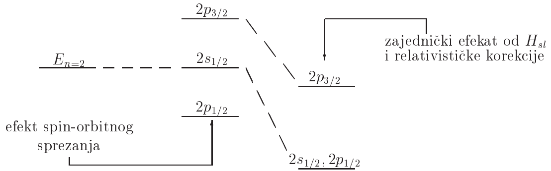
Slika 9.2: Cepanje energetskog nivoa E_{n=2} pri računanju fine strukture.
