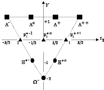
Slika 8.8: Hadronski K -supermultiplet.
