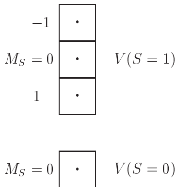
Slika 7.6: Razlaganje spinskog faktor prostora stanja \mathcal{H}_{12}^{(s)} dve čestice.
